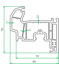
پروفیل باز شو دکوراتیو پنجره 563/02
