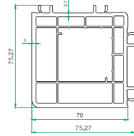
پروفیل اتصال ۹۰ درجه 563/10
