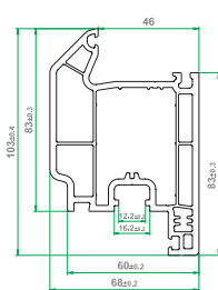
پروفیل باز شو در 507/04
