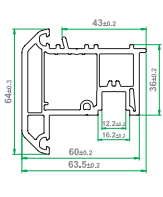
پروفیل میانی متحرک 507/05
