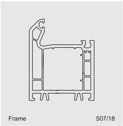
پروفیل قاب بلند
