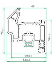
پروفیل باز شو دکوراتیو پنجره 507/02
