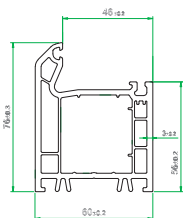
پروفیل قاب بلند 507/18
