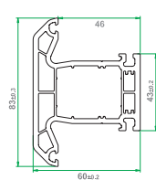
پروفیل میانی ثابت 507/03
