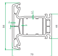
پروفیل میانی ثابت 563/03
