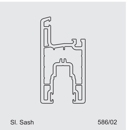
پروفیل باز شو کشویی
