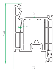
پروفیل باز شو در 563/15
