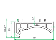
پروفیل آداپتور گرد 563/08
