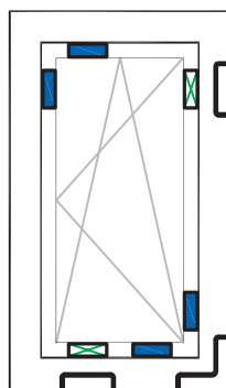
Tilt&turn window
